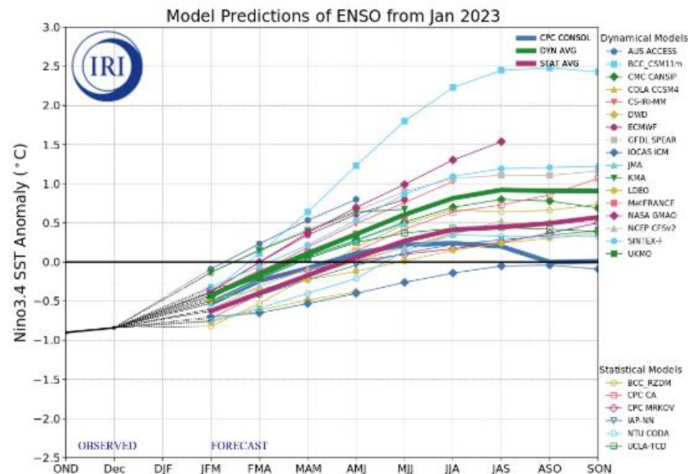
图15、不同模型对ENSO指数的预测（1月）
