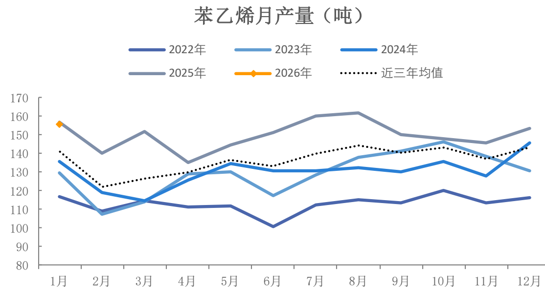
图12、苯乙烯产量
