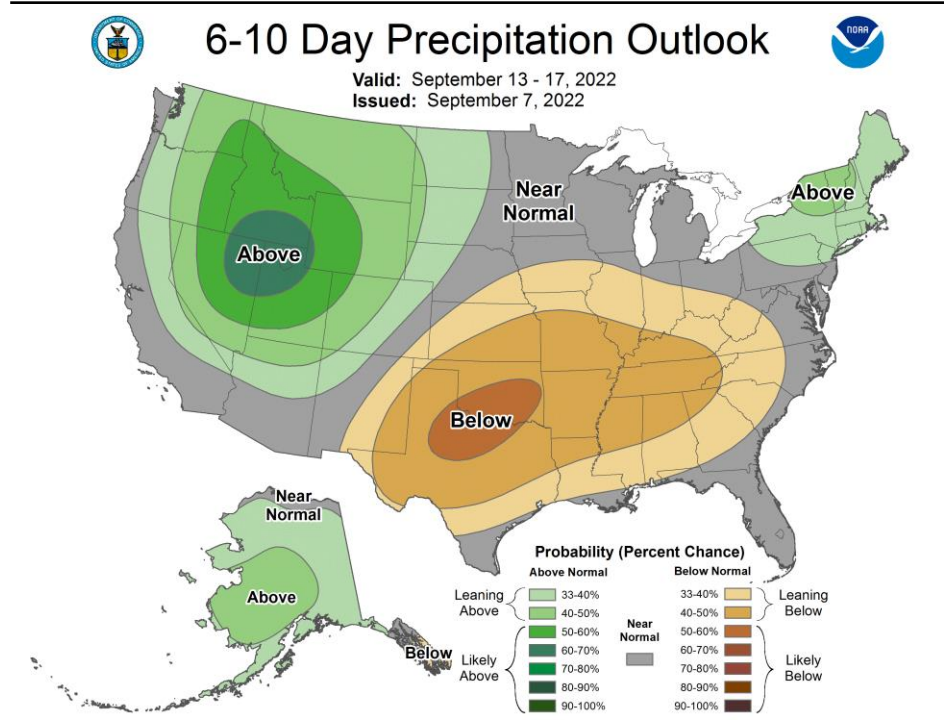
图8、0913-0917降水量前瞻
