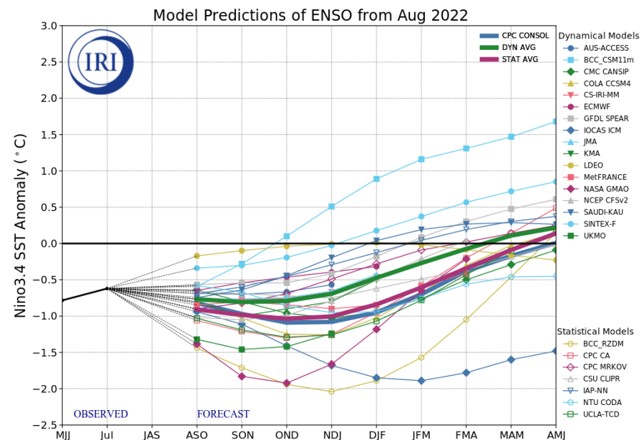
图21、不同模型对ENSO指数的预测
