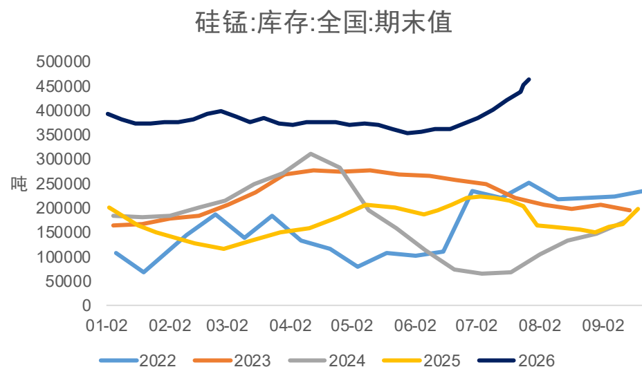
图9、硅锰库存
