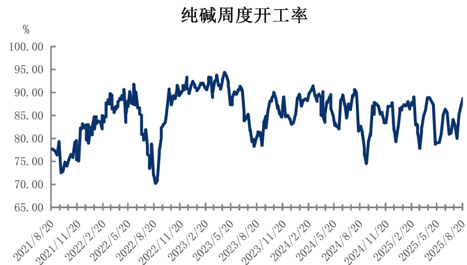
图12 国内纯碱装置产能开工率
