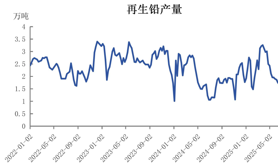
图9 再生铅产量
