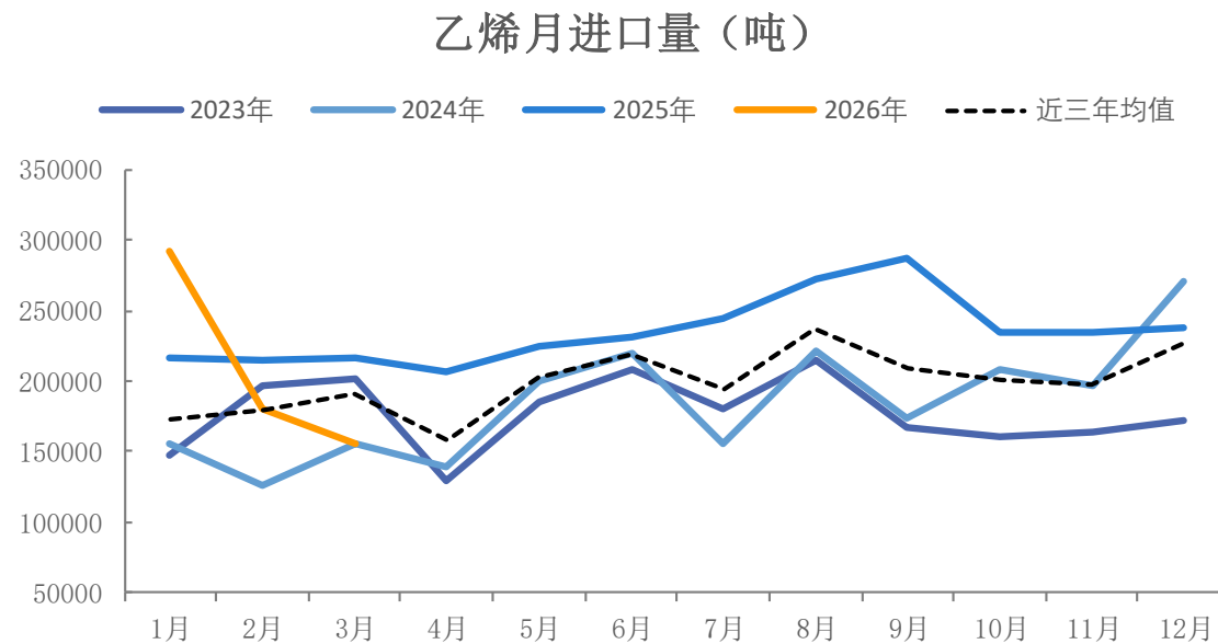
图10、乙烯进口量
