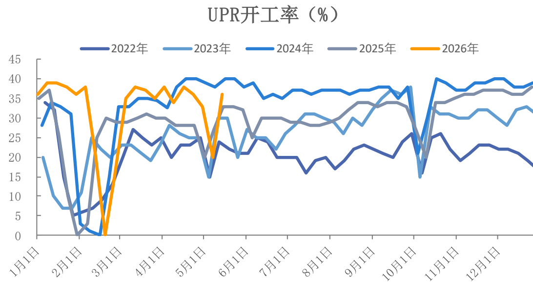
图19、UPR开工率
