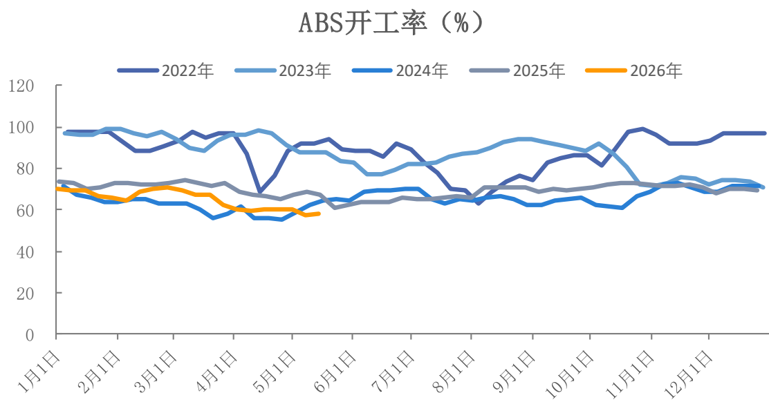
图18、ABS开工率
