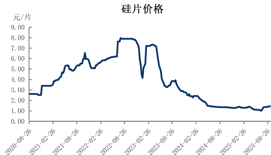
图17 硅片价格
