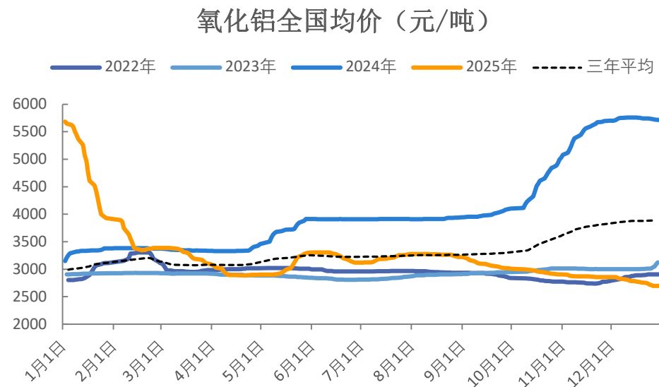
图21、氧化铝价格
