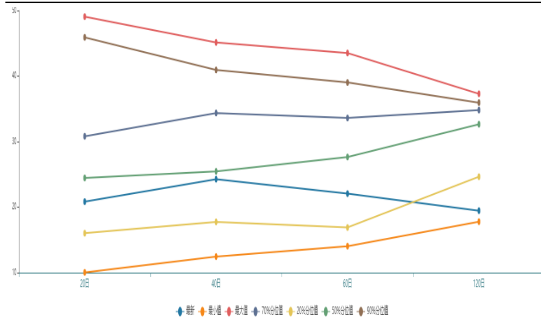
图25、波动率锥
