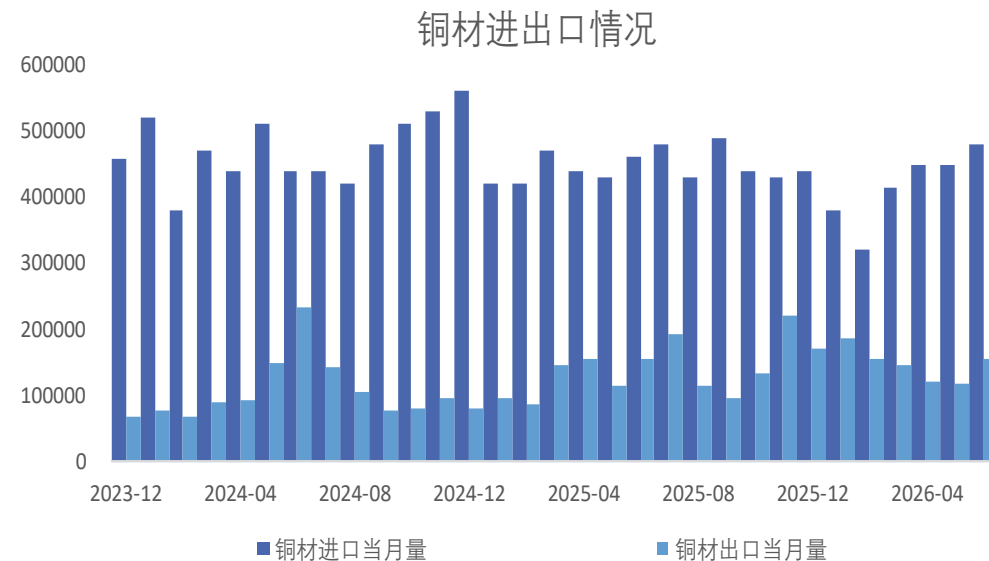
图20、铜材进出口
